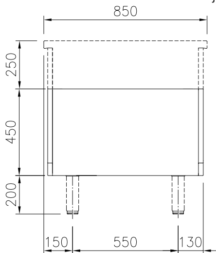
Boven aanzicht
